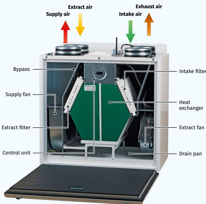
KOMFORT EC SB
